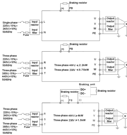
3-3 diagramm Főáramkör kapcsolási rajza
